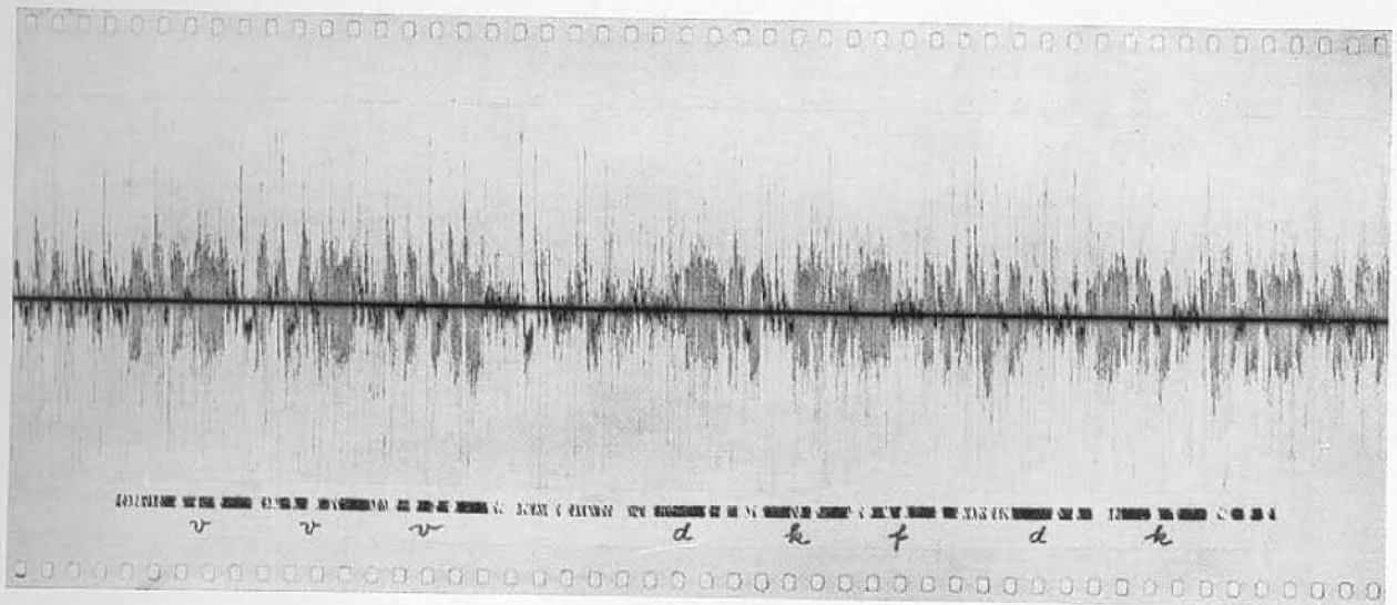
Abb. 9: Oszillogramm der Empfängerausgangsspannung mit zugehörigem Empfangsstreifen bei gestörtem Funkempfang. Die Störampplitude beträgt ein Mehrfaches der Zeichenamplitude. Die Störungen werden zwischen den Morsezeichen als Punkte abgebildet.
