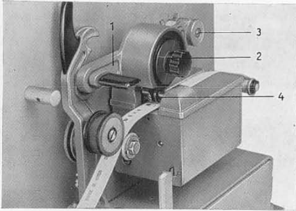
Abb. 3: Schreibrad mit Farbrolle und Papiertransport.
