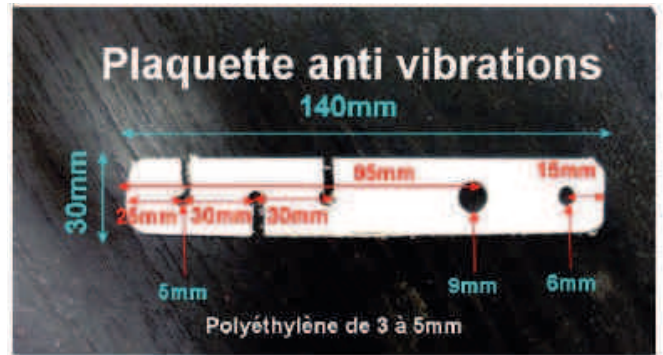
Fabrication de la plaquette anti-vibrations
