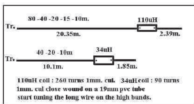
Schéma des deux versions d'antennes
