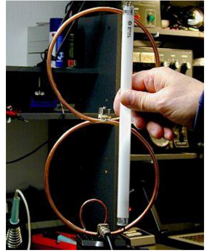
Zero horizontal polarisation.
