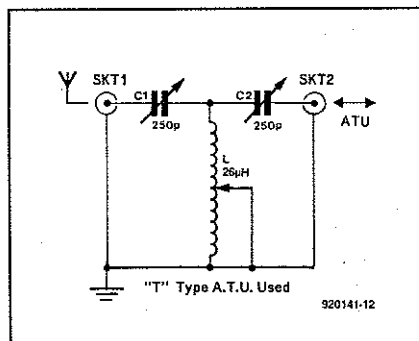
Fig. 2. Type 'T' ATU used.
