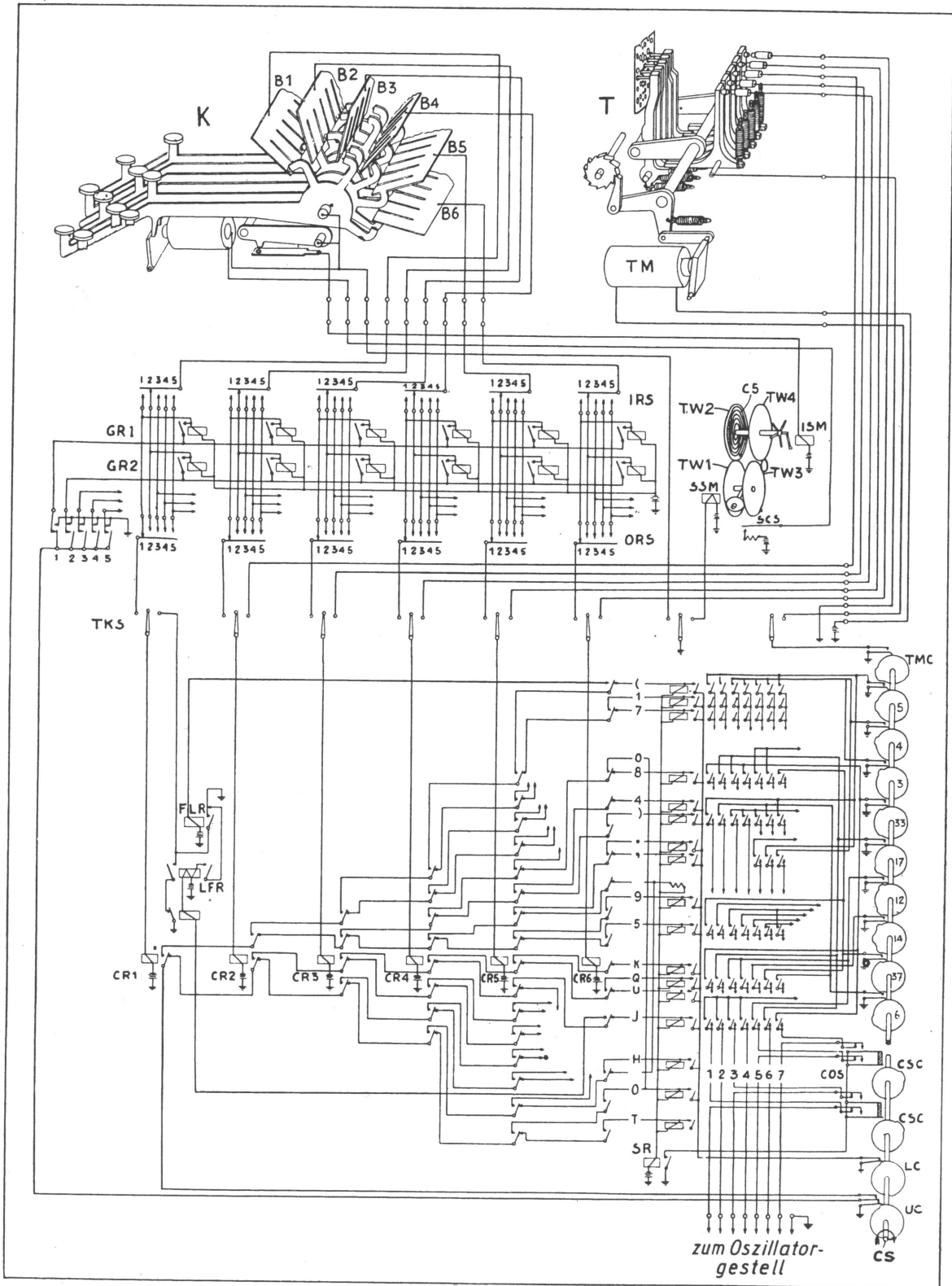
Bild 3. Schaltschema des Senders; a) zum Oszillatorgestell.
