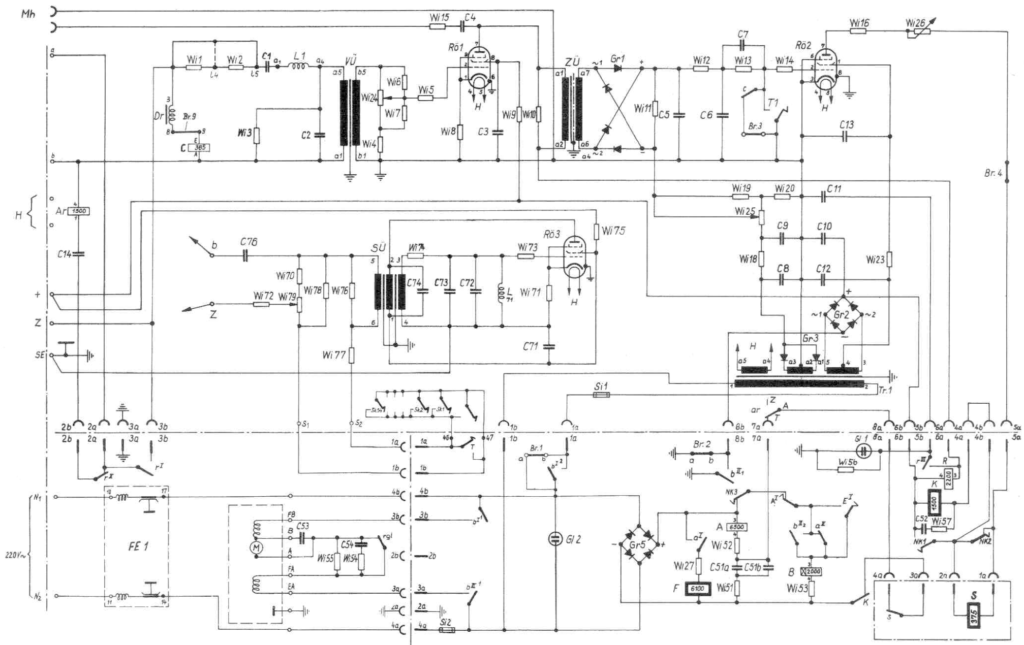
Hellschreiber T typ72a
